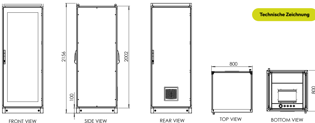
Technische Zeichnung
